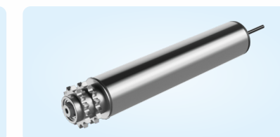
直径76mm，圆柱形 温度范围 -40℃~ 55℃ 页码 18
