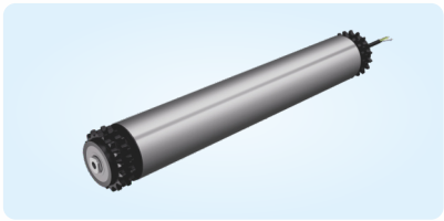
两端双链轮滚筒 温度范围 -40℃~55℃ 页码22
