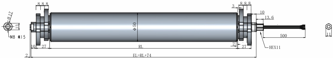
动力滚筒
