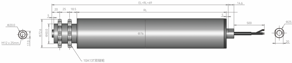
Φ76/80/89mm 系列尺寸图
