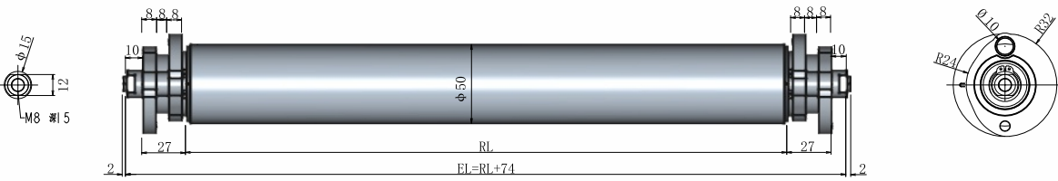
从动滚筒
