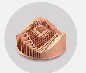
铜打印结构 打印材料: 纯铜 最小壁厚0.1mm 最小孔径0.3
