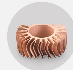
散热器 打印材料: 纯铜 散热器内部复杂螺旋流道 散热片最小壁厚0.5mm
