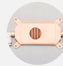
液冷板 打印材料: 纯铜
