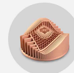
铜打印结构 打印材料: 纯铜 最小壁厚0.1mm 最小孔径0.3
