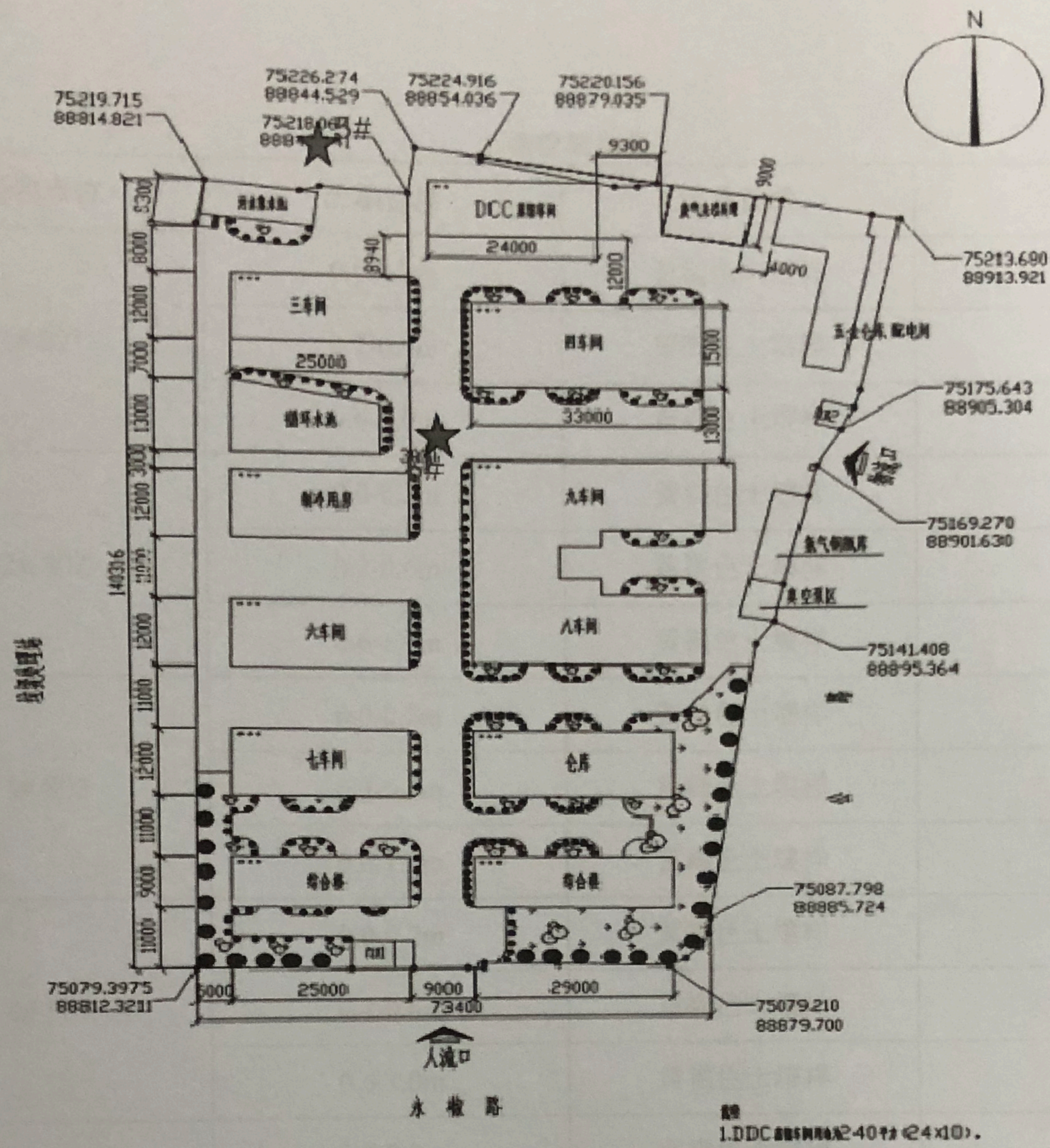
厂区平面图 1:800
